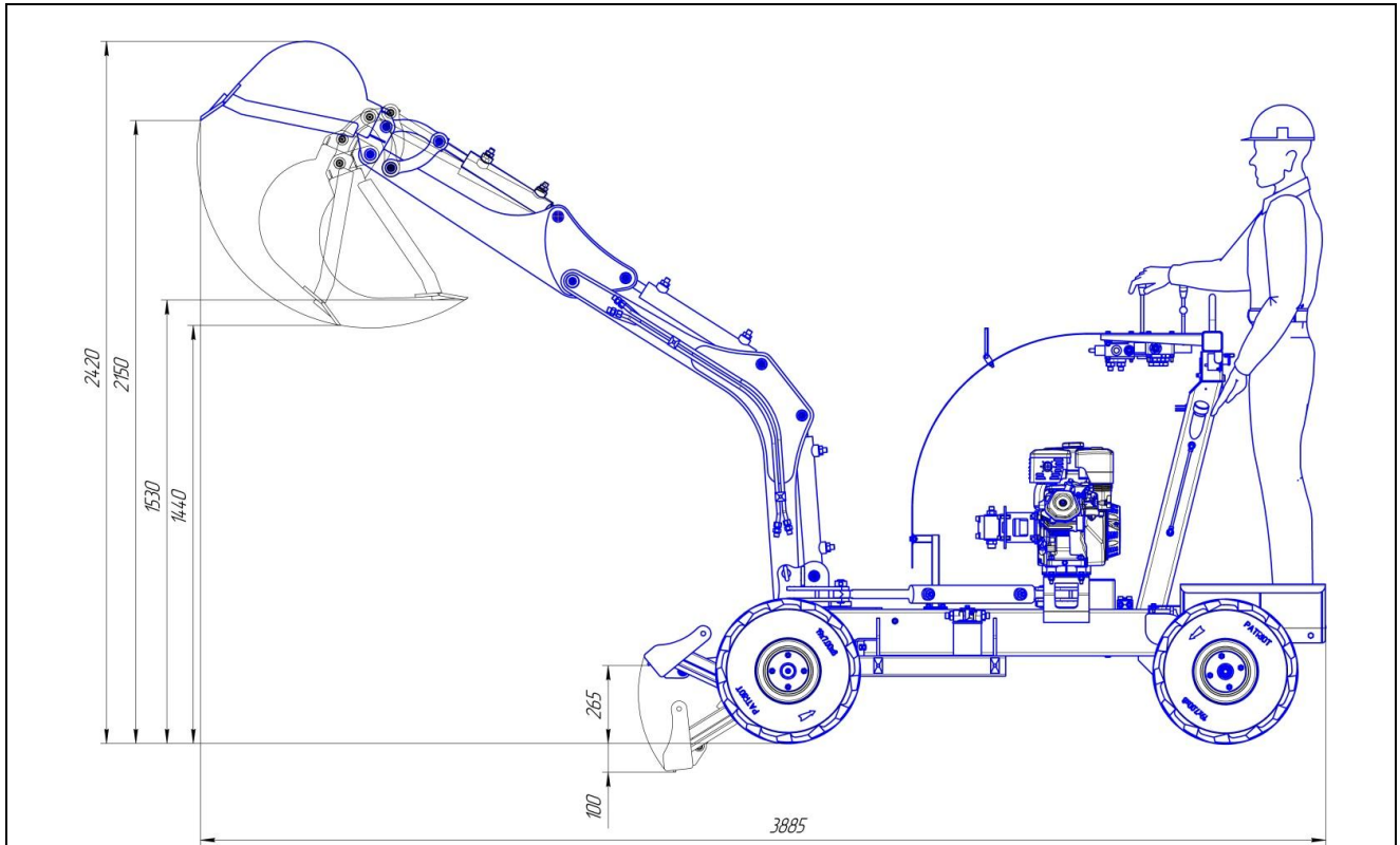
Параметрическая схема. Положения ковша и отвала.
