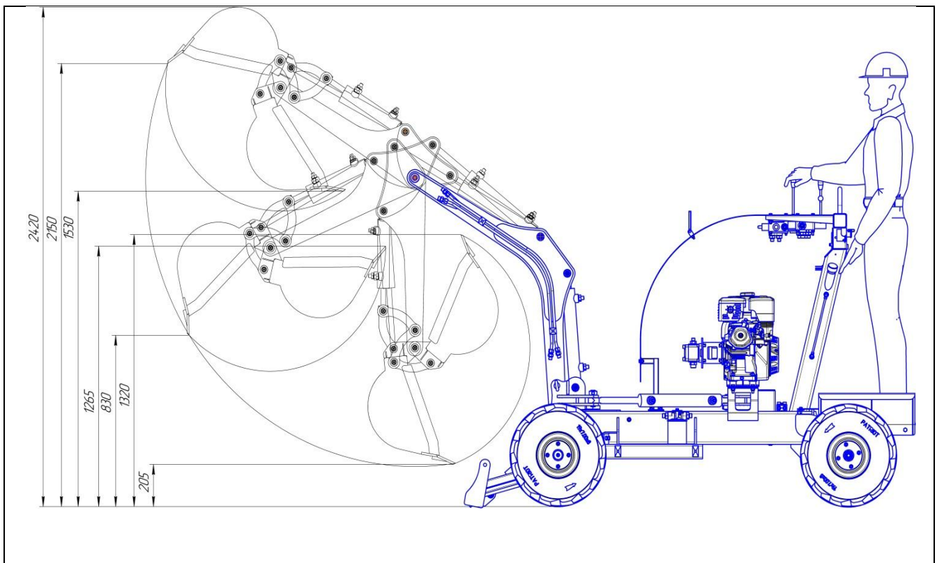
Параметрическая схема. Положения ковша и рукояти
