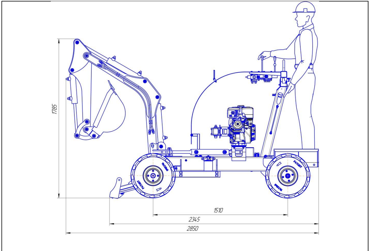
Транспортное положение экскаватора. Вид слева.
