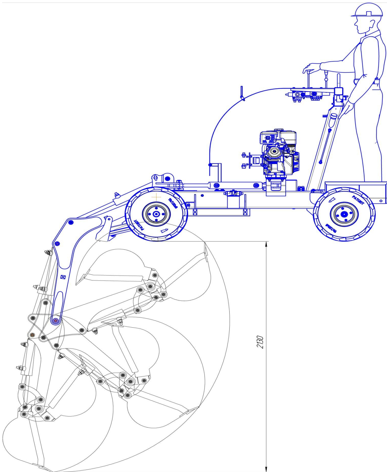
Параметрическая схема. Положения ковша, рукояти и стрелы.
