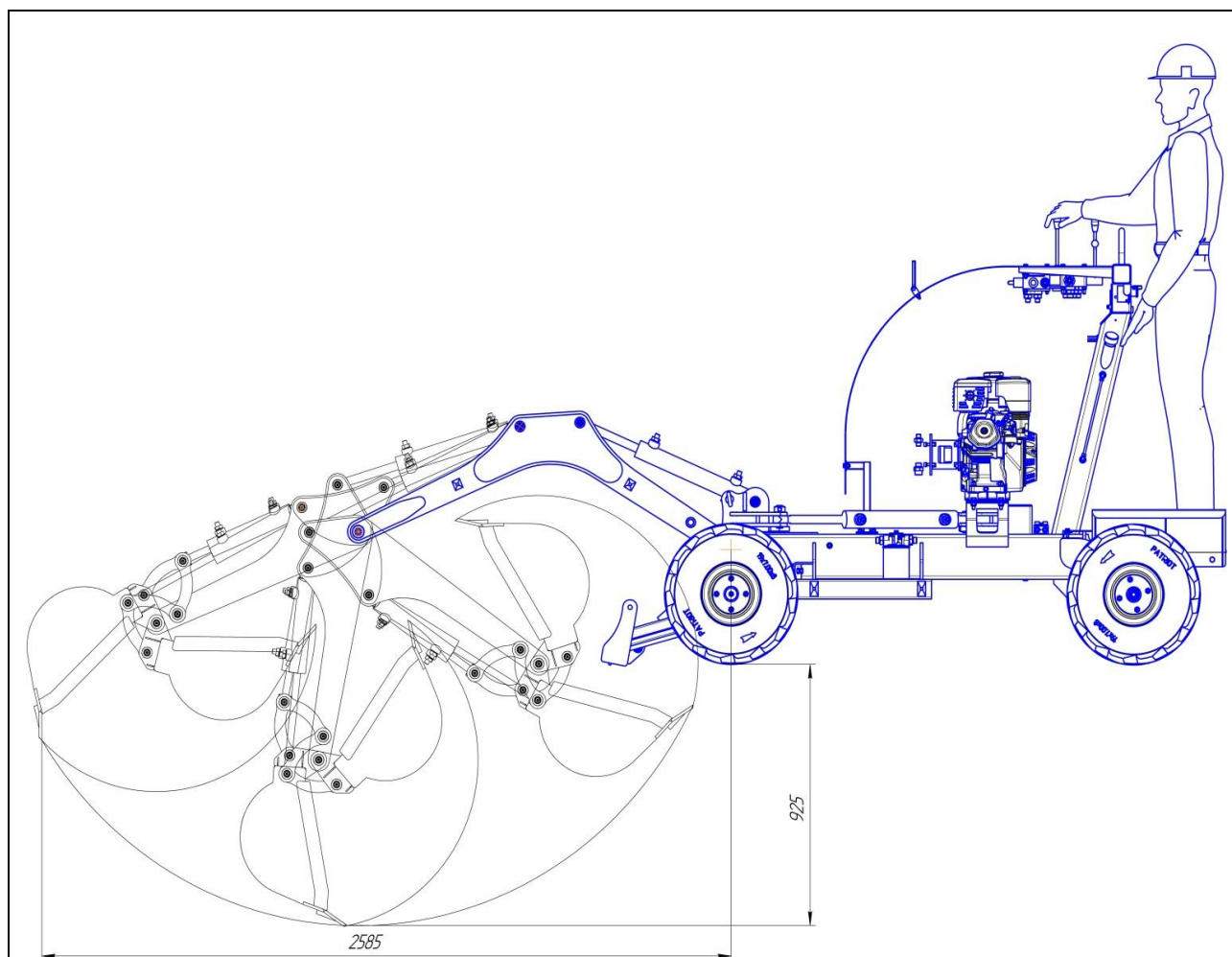
Параметрическая схема. Положения ковша, рукояти и стрелы.
