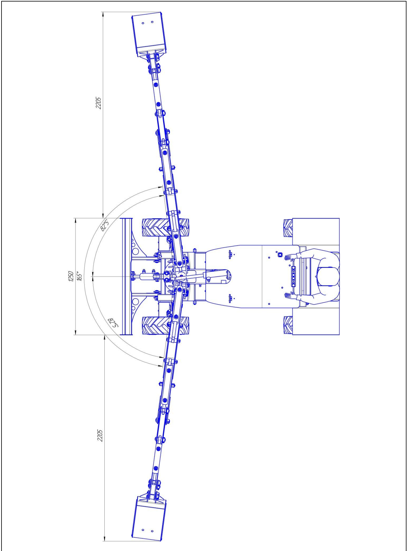
Рабочее положение экскаватора. Максимальные углы поворота стрелы.
