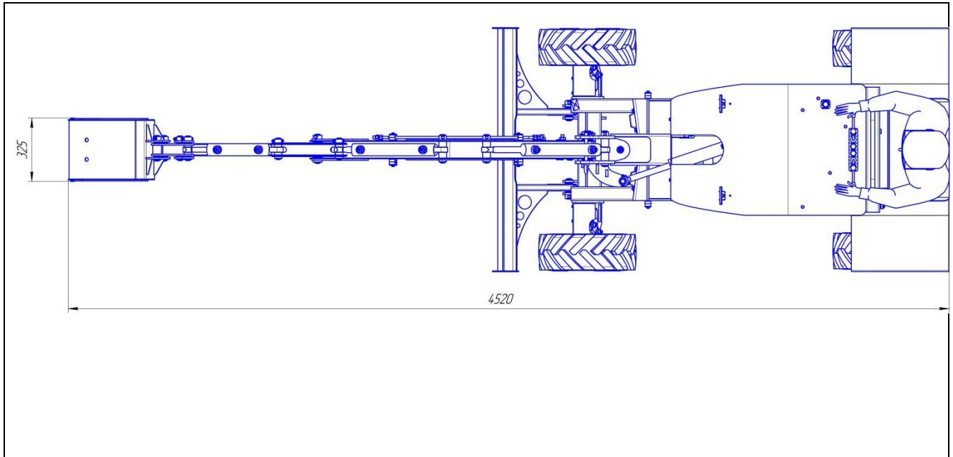
Рабочее положение экскаватора. Максимальный вылет стрелы. Вид сверху.
