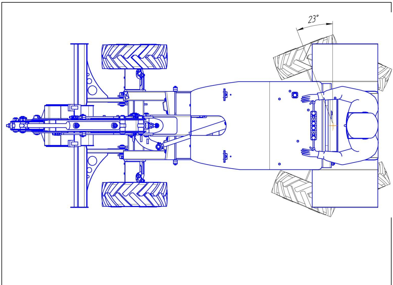
Углы поворота заднего моста.
