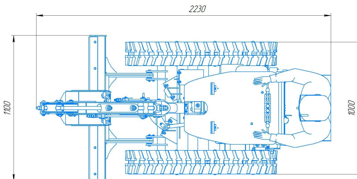
Транспортное положение экскаватора. Вид сверху
