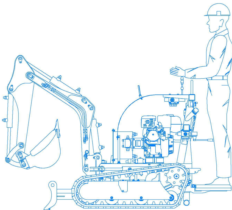
Транспортное положение экскаватора. Вид слева.
