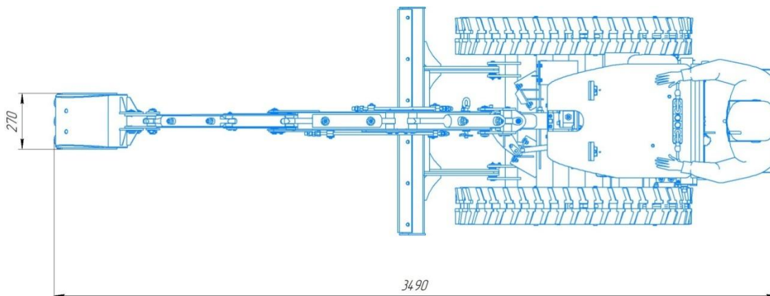
Рабочее положение экскаватора. Максимальный вылет стрелы. Вид сверху.
