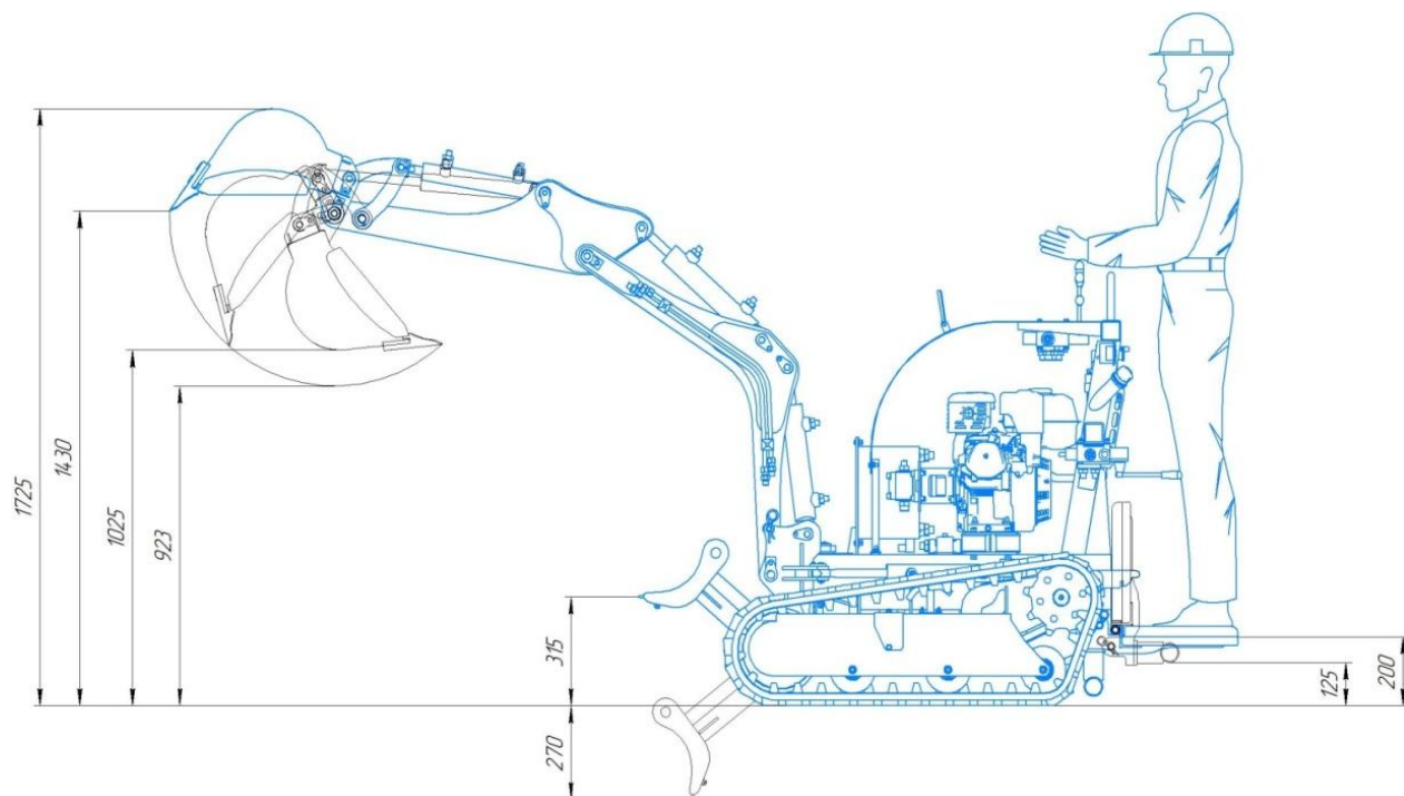
Параметрическая схема. Положения ковша и отвала. Рис. 5
