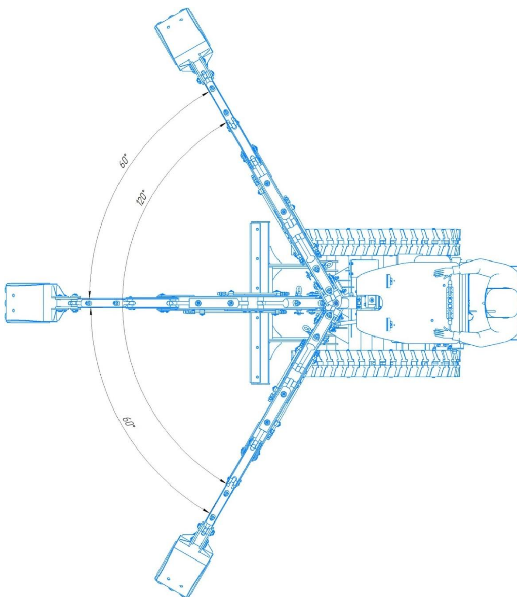
Рабочее положение экскаватора. Максимальные углы поворота стрелы
