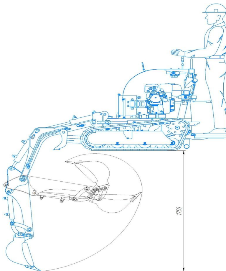
Параметрическая схема. Положения ковша, рукояти и стрелы.
