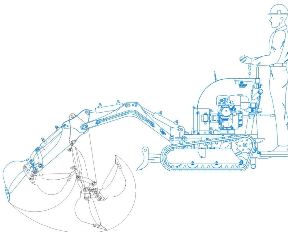
Параметрическая схема. Положения ковша, рукояти и стрелы.
