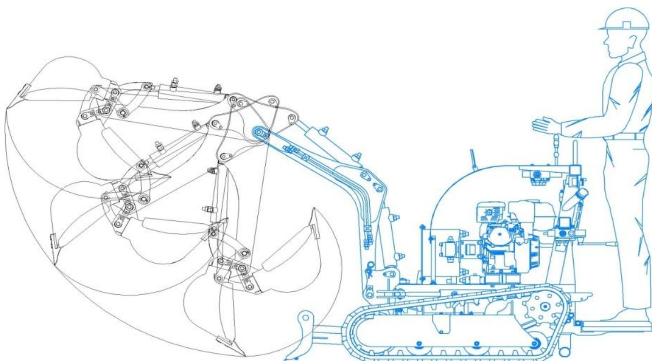
Параметрическая схема. Положения ковша и отвала. Рис. 5
