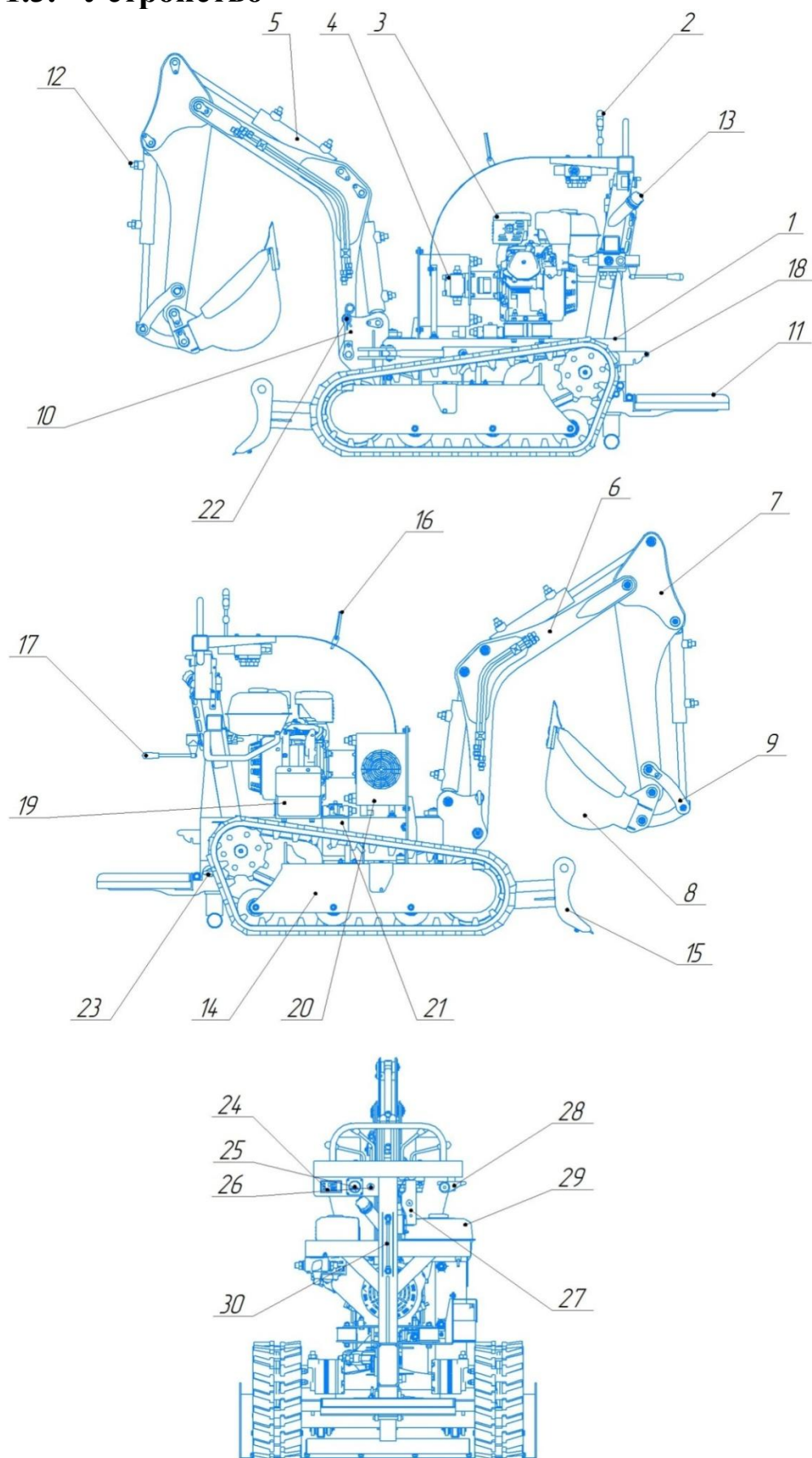
Устройство мини экскаватора. Рис.9
